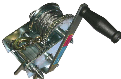
Лебедка ручная стационарная с ручным тормозом. Грузоподъемность - 1100кг, длина троса - 10м, диаметр - 6мм
